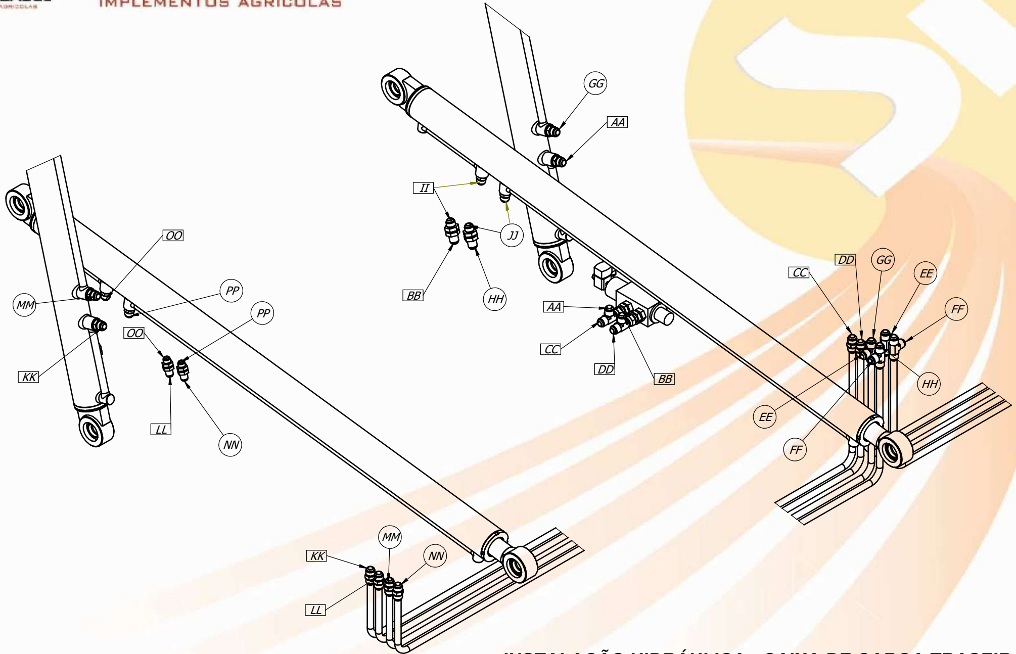
INSTALAÇÃO HIDRÁULICA - CAIXA DE CARGA TRASEIRA
